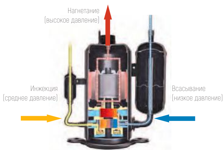
ДВУХСТУПЕНЧАТЫЙ DC - ИНВЕРТОРНЫЙ КОМПРЕССОР
